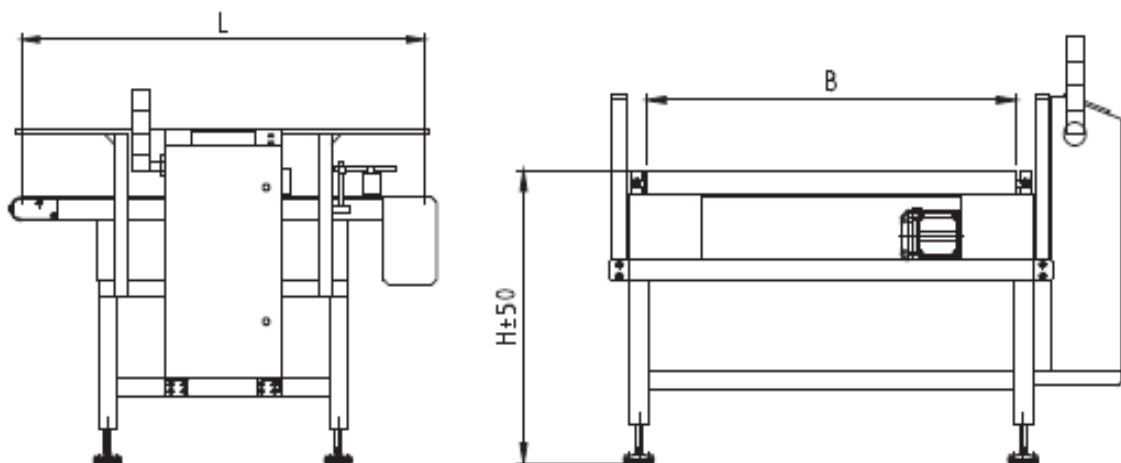
Z001 自动检重秤技术参数 单位：mm
